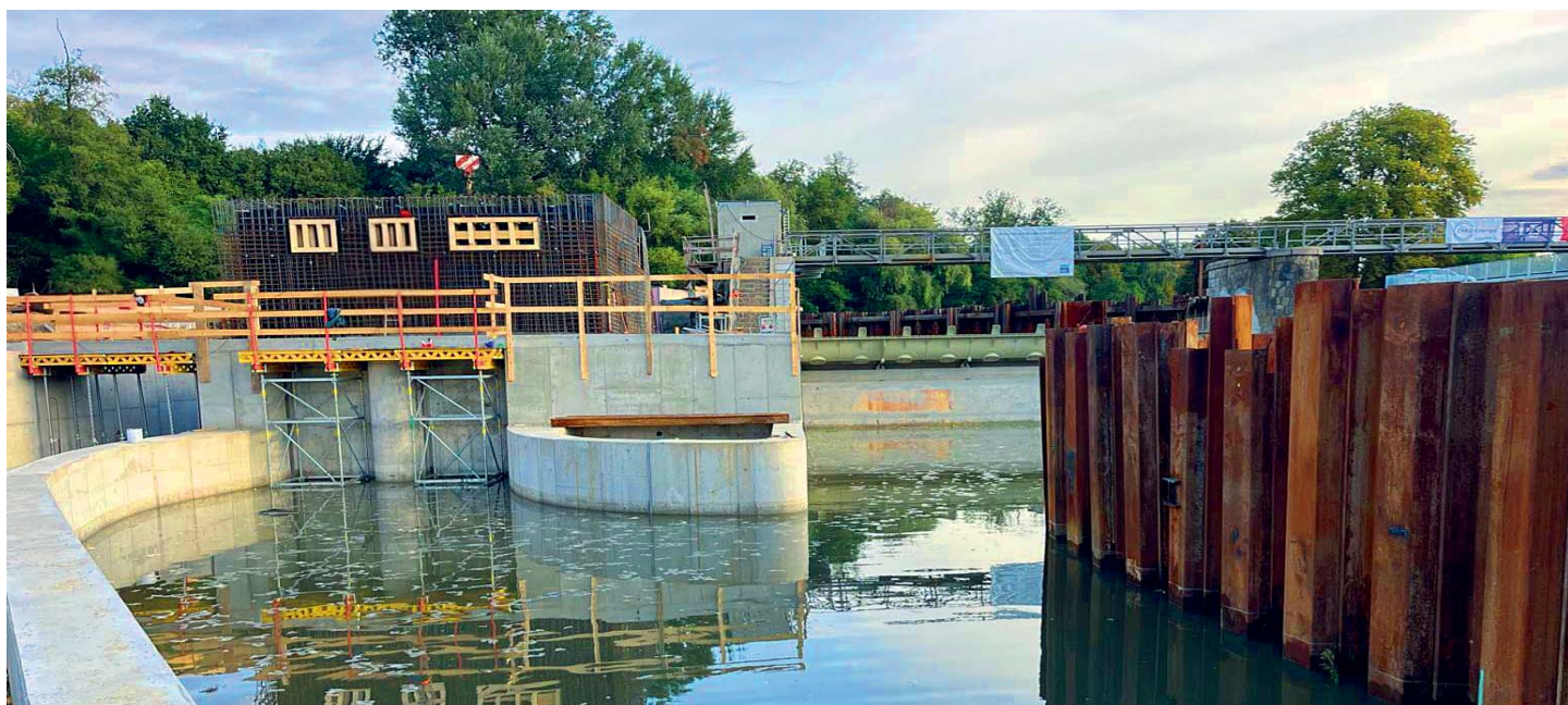
Pohled na zatopený výtok z MVE při zahájení demontáže jímky na spodní vodě
