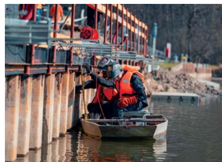
Svařovací práce na nábrežní hraně probíhaly z vody
